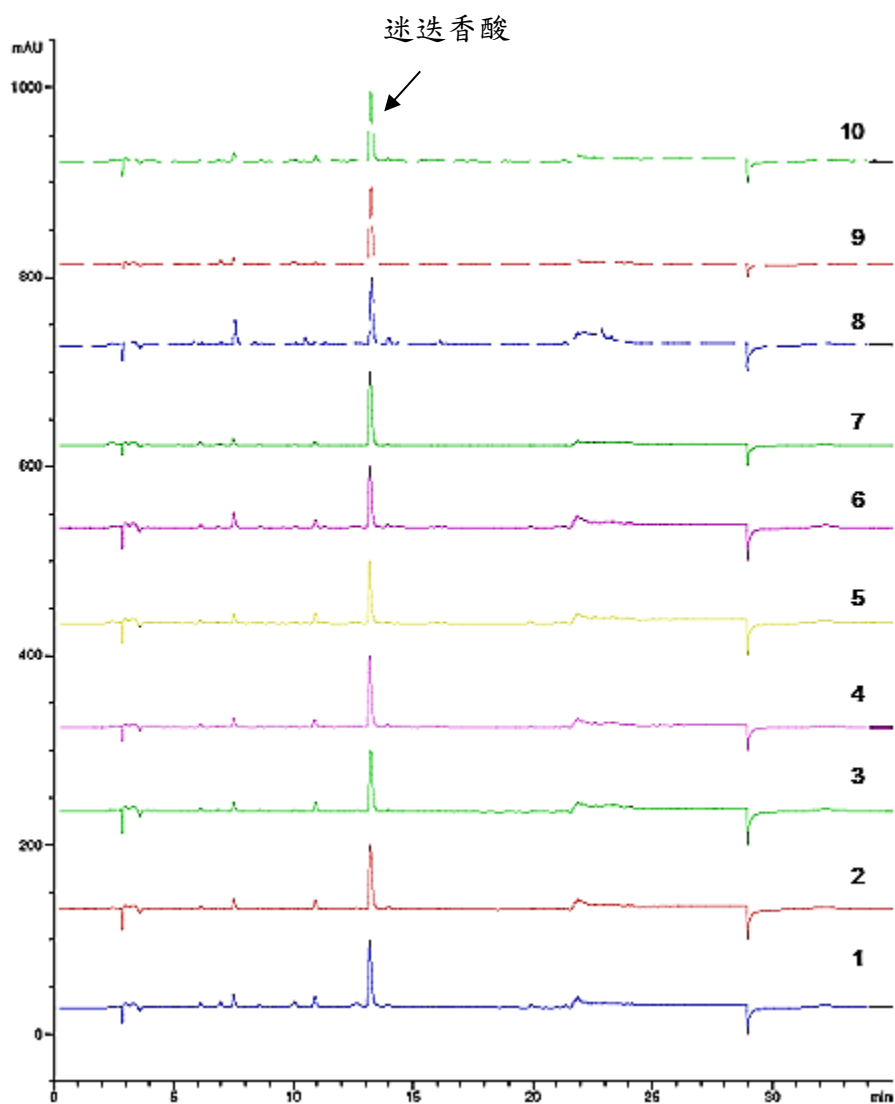
圖六、10 批紫蘇梗藥材之 HPLC 指紋圖譜
