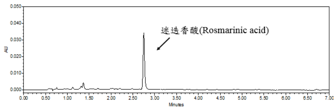
圖八、市售紫蘇梗檢品之 UPLC 層析圖
