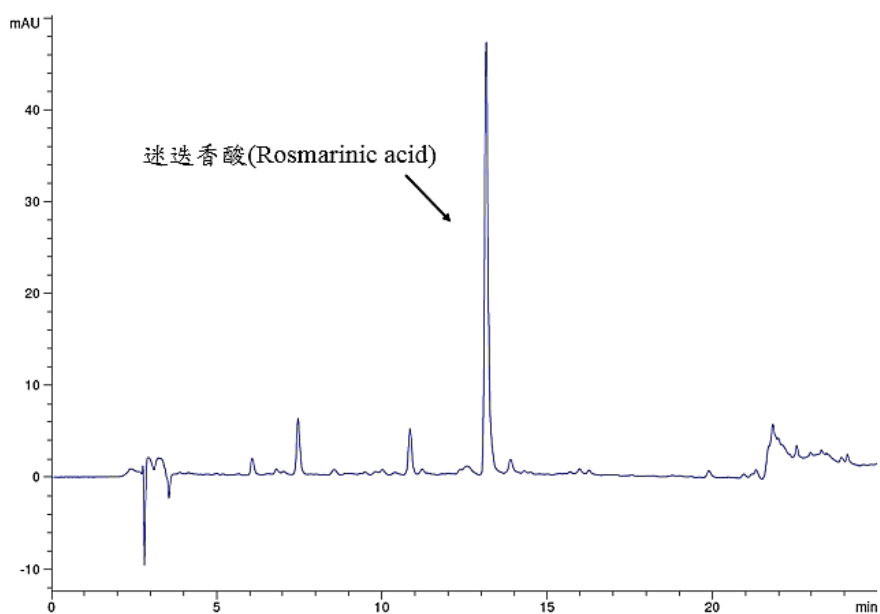
圖二、市售紫蘇梗檢品之 HPLC 層析圖
