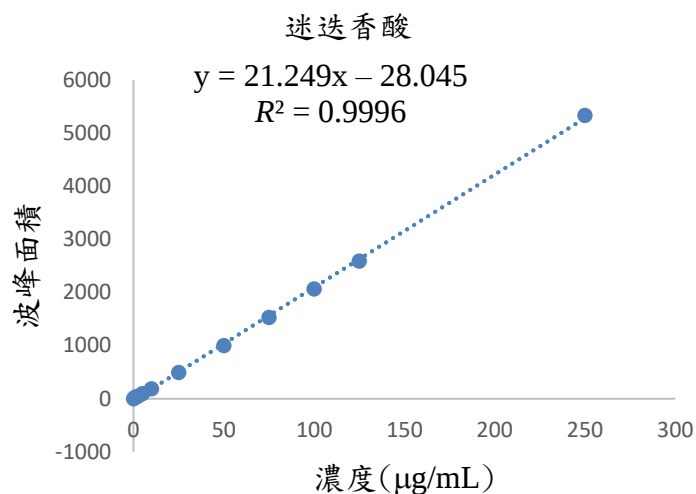
圖三、迷迭香酸之檢量線圖
