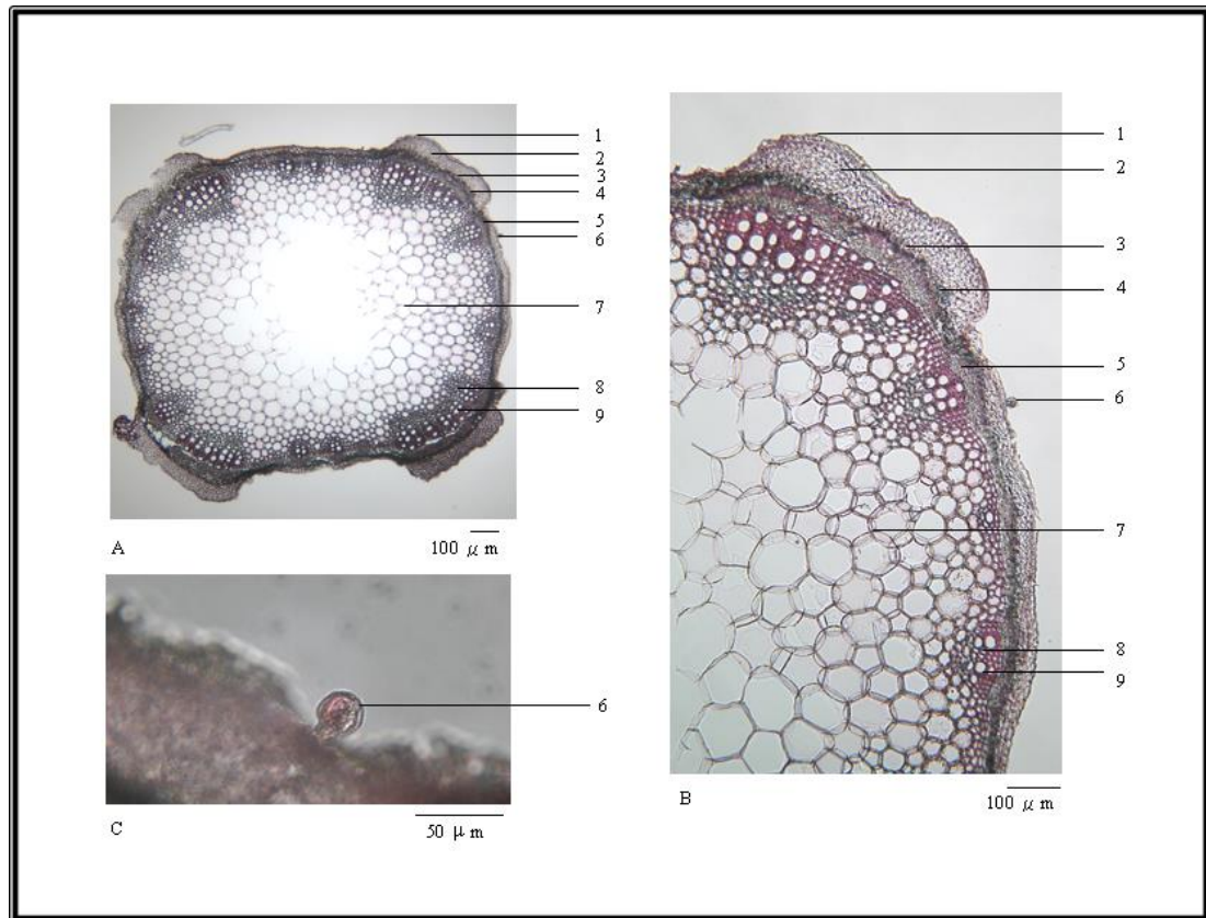
圖 2 紫蘇梗橫切面顯微特徵圖
