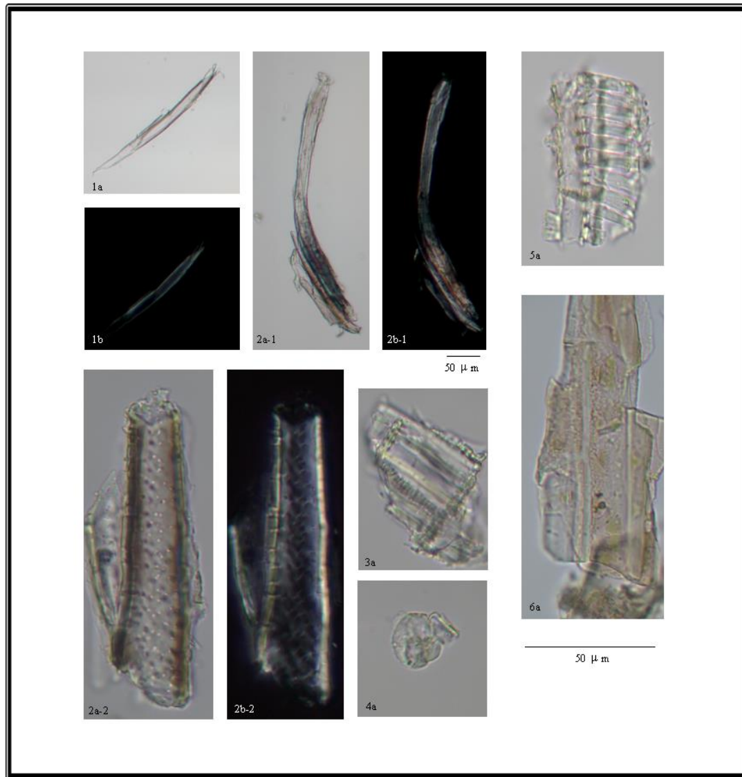
圖 3 紫蘇梗粉末顯微特徵圖
